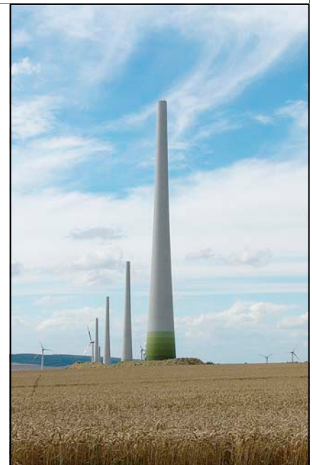
Wegen Anlagen- und UW-Schaden standen diese 6 Anlagen über 2 Wochen still
